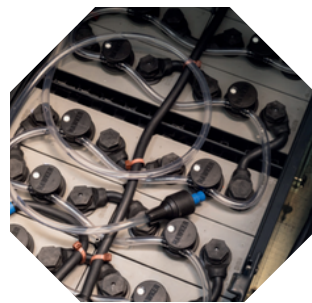
Gekapselte 24V Antriebsbatterie im Spezialtrog sichert höchsten Schutz.
